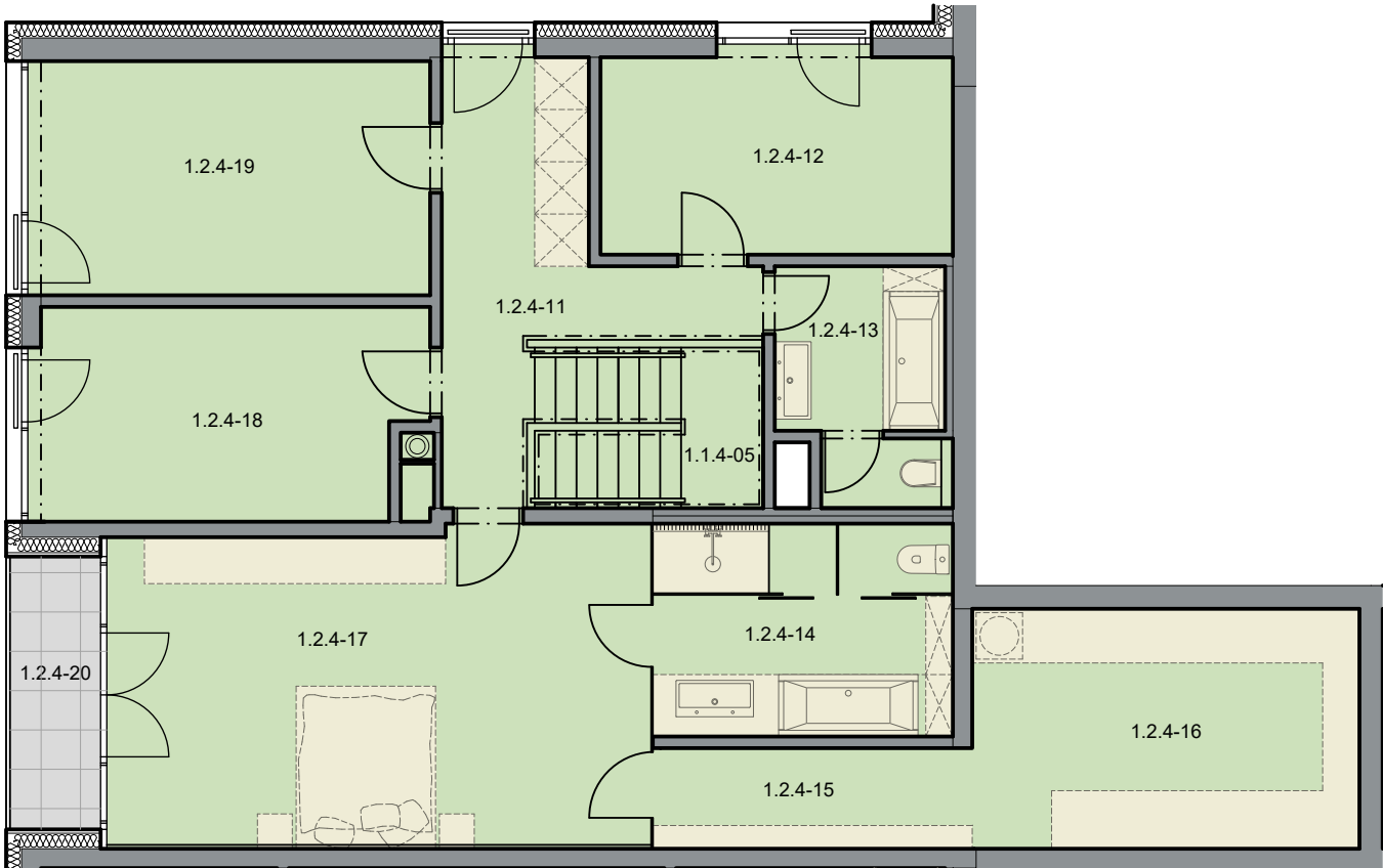
PŮDORYS 2NP 1:100
